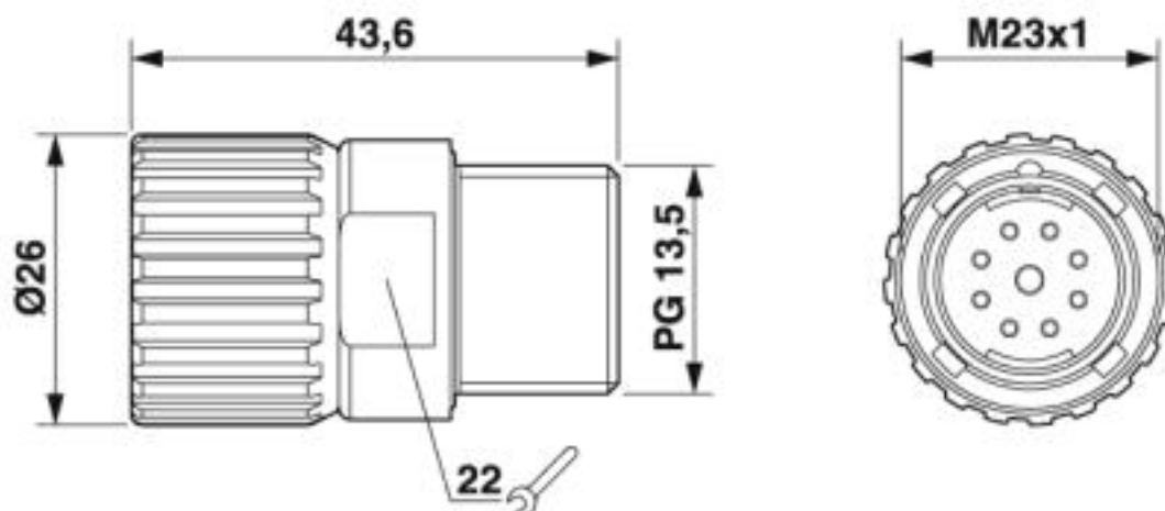
Disegno quotato
