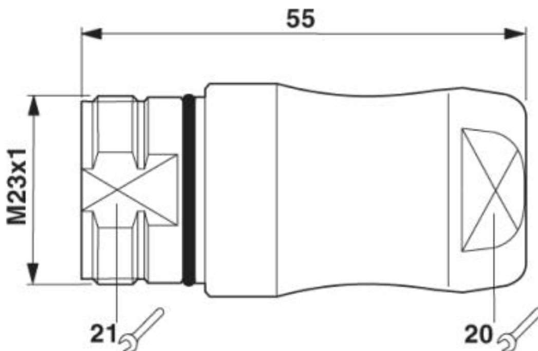
Disegno quotato
