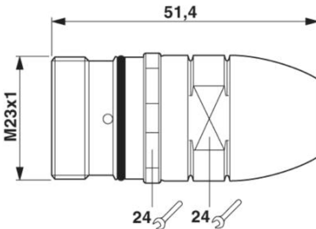
Disegno quotato
