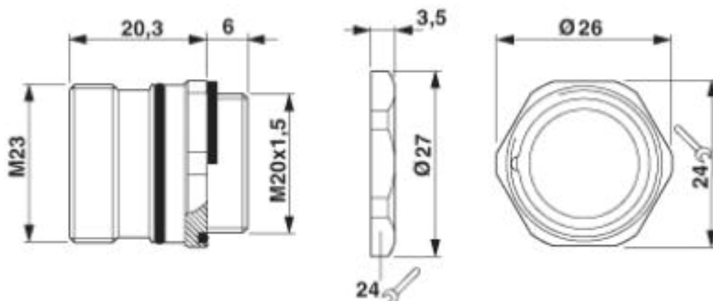
Disegno quotato
