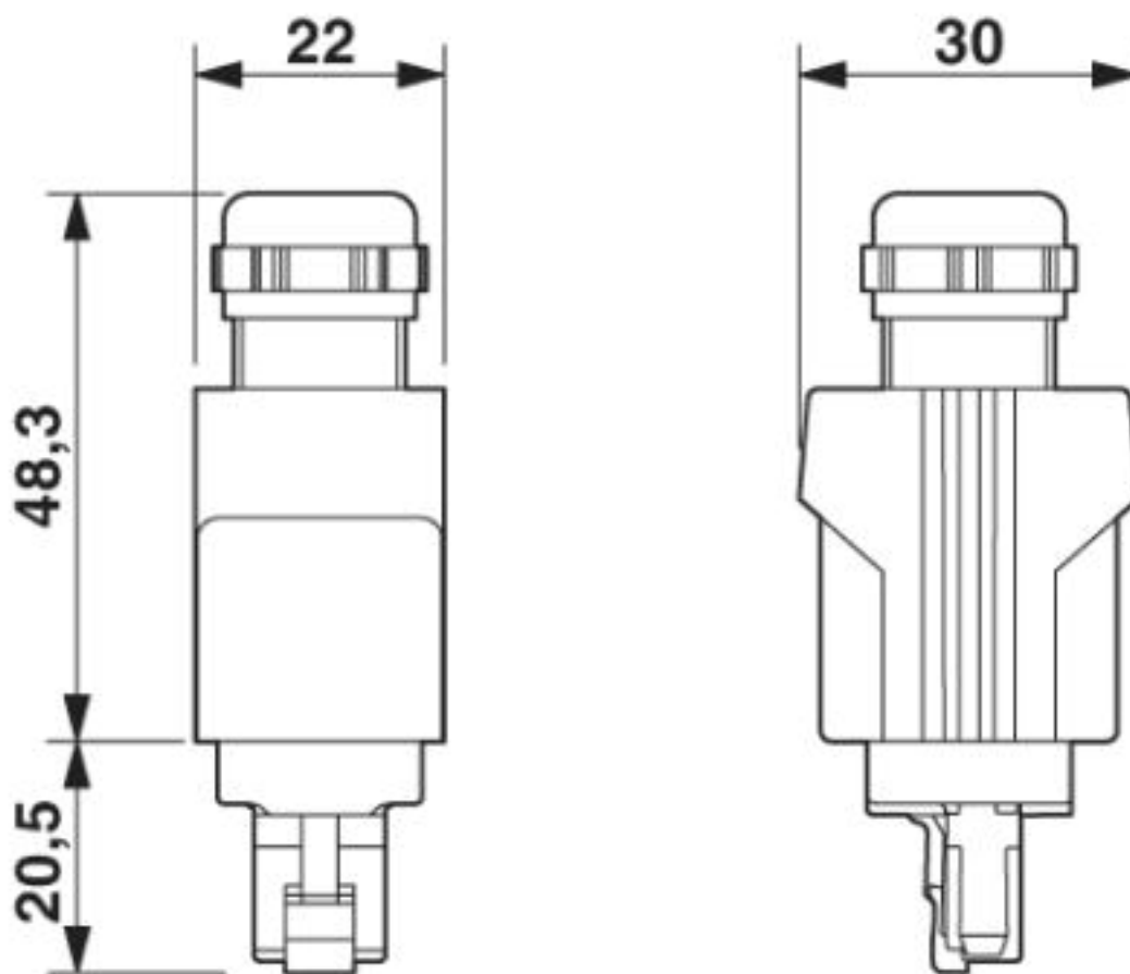
Connettore push-pull RJ45 IP65/67
