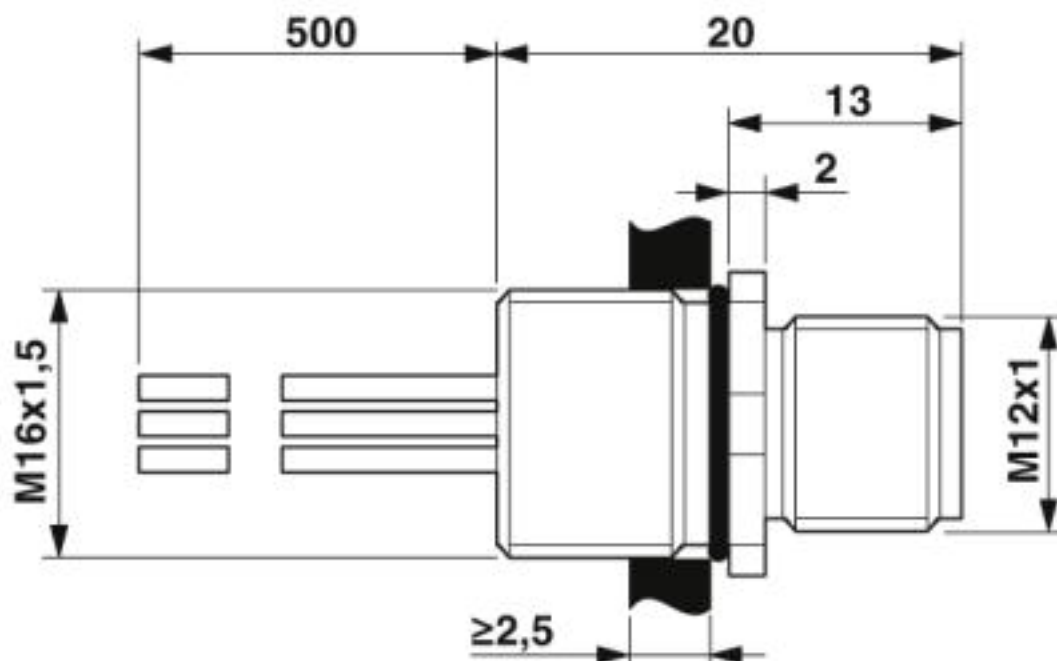
Disegno quotato
