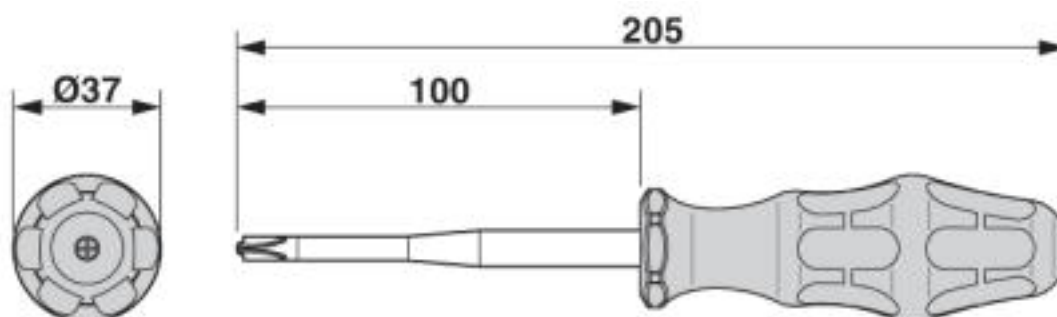
Disegno quotato
