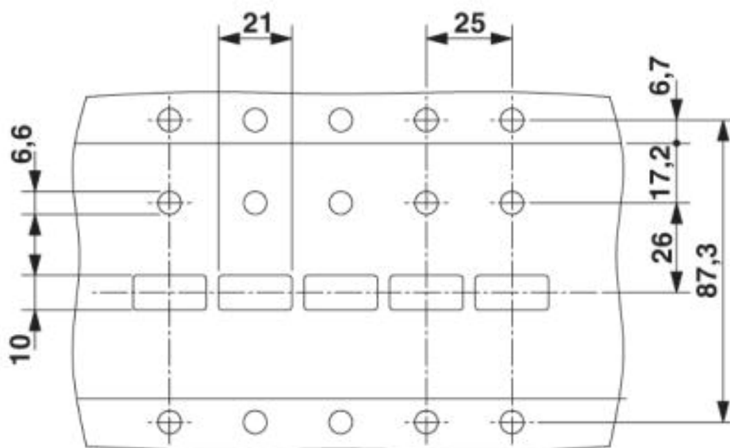
Disegno quotato
