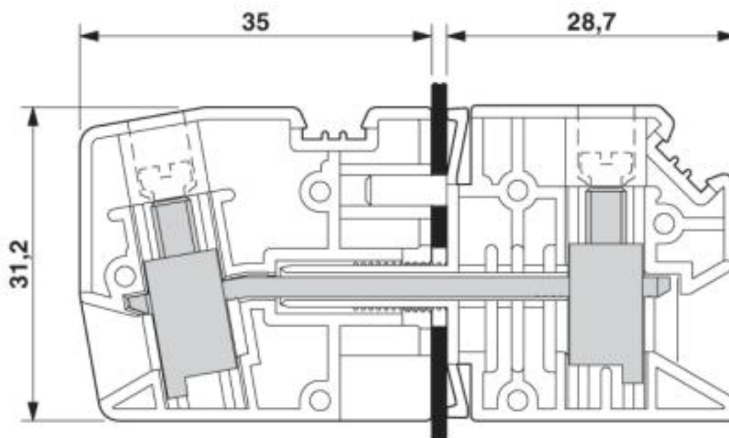
Disegno quotato
