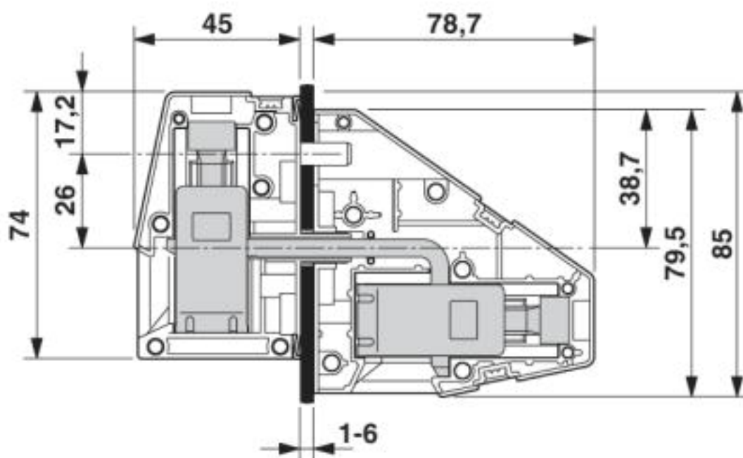
Disegno quotato
