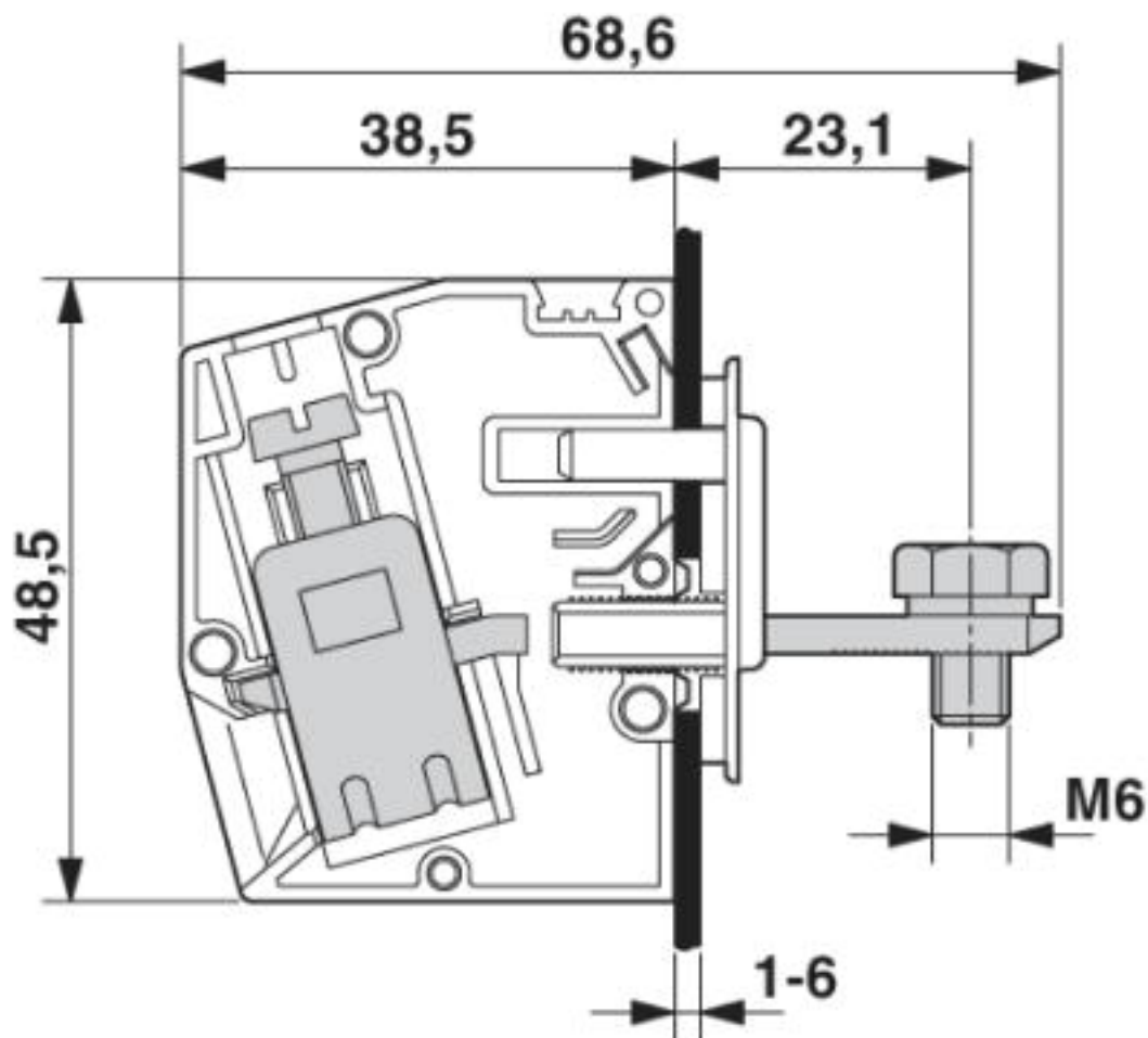
Disegno quotato
