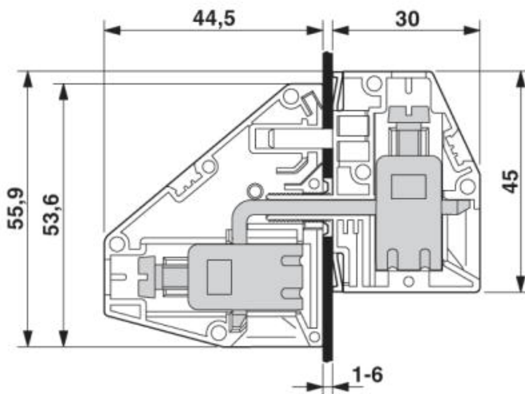
Disegno quotato
