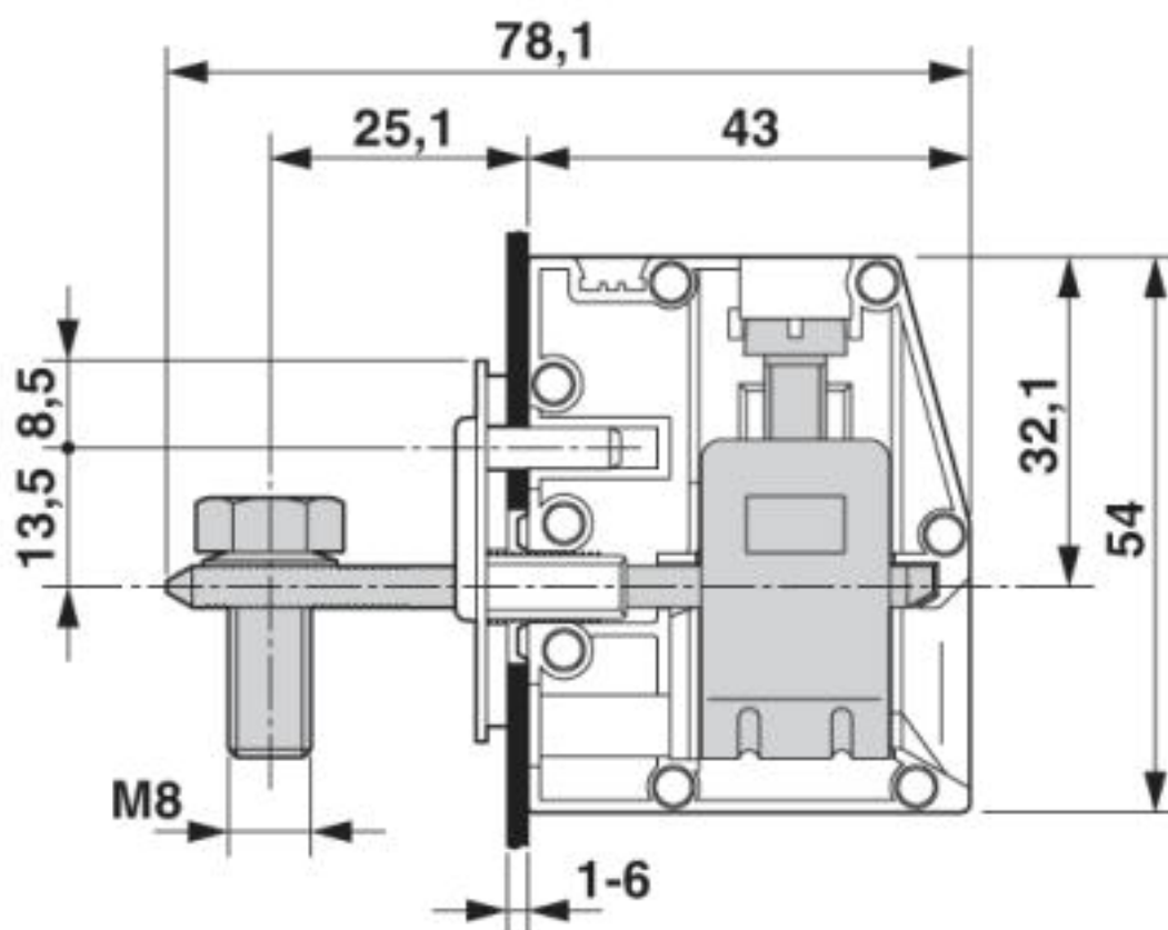
Disegno quotato
