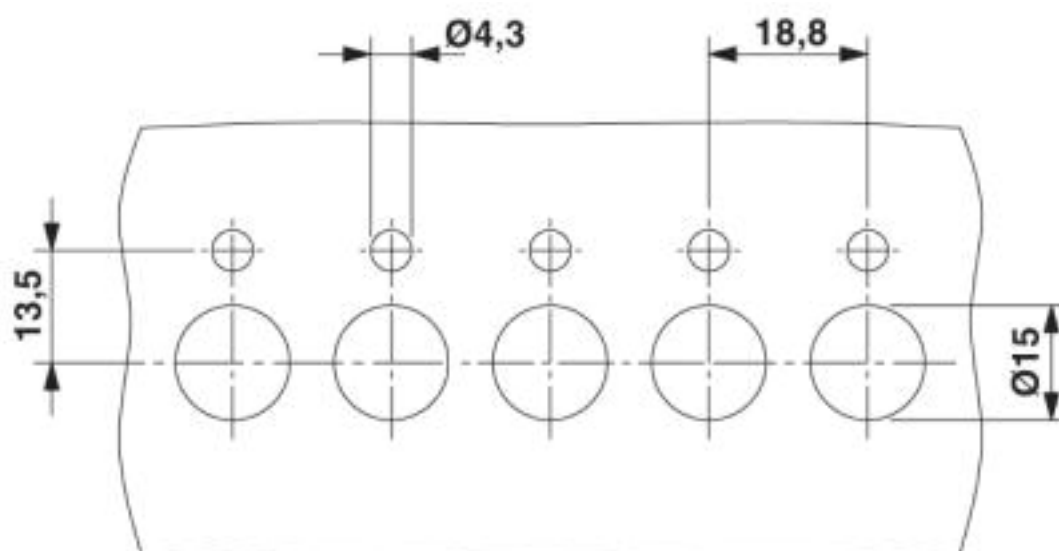
Disegno quotato
