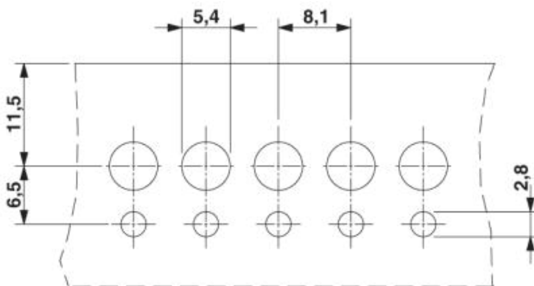
Disegno quotato
