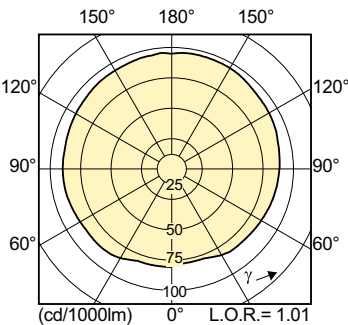
Light Distribution Diagram - MASTERCoulour CDM-T MW eco 230W/842 E40
