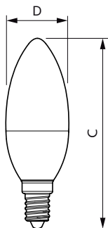
Candle B35 5-40W 470lm 6500K E14 ND FR
