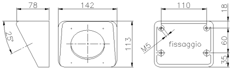
Supporto isolante (per finestra tipo "a")
