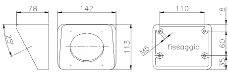
Supporto isolante (per finestra tipo "a")
