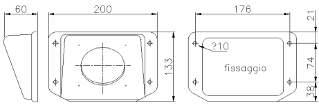
Supporto in lega di alluminio (per finestra tipo "F5")
