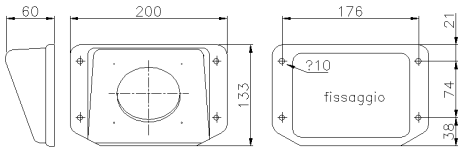
Supporto in lega di alluminio (per finestra tipo "F5")
