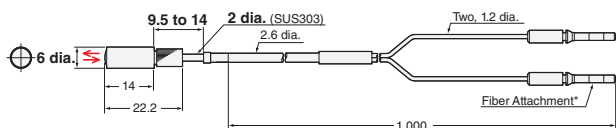
25-B E32-C42 1M (No Cutting) + E39-F17
