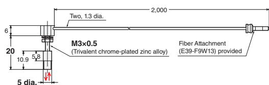
25-D E32-C21N 2M (Free Cutting) + E39-F3C
