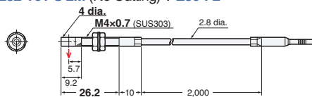
33-I E32-T61-S 2M (No Cutting) + E39-F2
