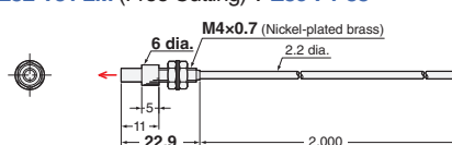
33-J E32-T51 2M (Free Cutting) + E39-F1-33
