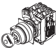
A22NK-2M□-01□A-G
