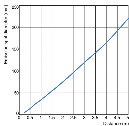
E3S-DB□□1(T)
