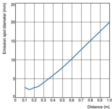
E3S-DB□□2(T)
