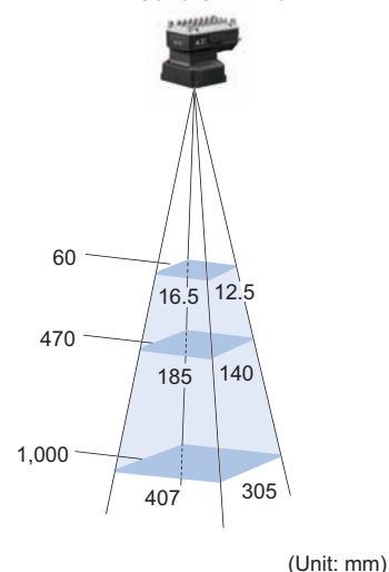
FHV7X-C016-S12-W-01
