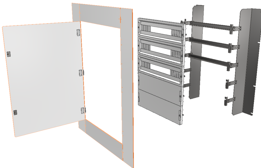
Sistema di allestimento quadri mediante telaio porta apparecchiature modulari
