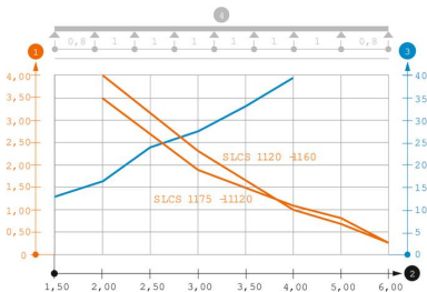
Diagramma di carico passerella tipo SLCS 110
