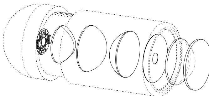
WR0301 - Accessory for positioning filters / Accessorio per posizionamento filtri
