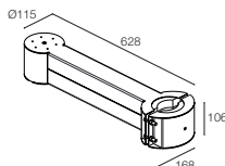
WP1005N - Black / Nero Arm for pole mounting / Braccio per attacco a palo
