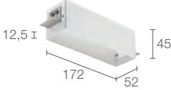
WC8705 - Bianco WC8705N - Nero Cassaforma per installazione arretrata su soffitto in cartongesso (opzionale) (Bitpop 4.1)
