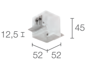
WC8703 - Bianco WC8703N - Nero Cassaforma per installazione arretrata su soffitto in cartongesso (opzionale) (Bitpop 1.0)
