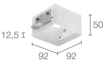
WC8704 - Bianco WC8704N - Nero Cassaforma per installazione arretrata su soffitto in cartongesso (opzionale) (Bitpop 2.2)
