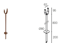
WP1002T Picchetto con staffa per installazione a terra - h 800 mm - cor-ten
