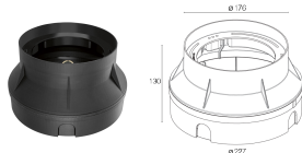
WCA03 Cassaforma
