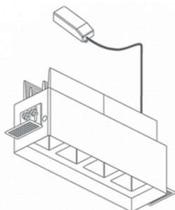
Installazione arretrata con cassaforma
