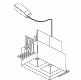
Installazione arretrata con cassaforma
