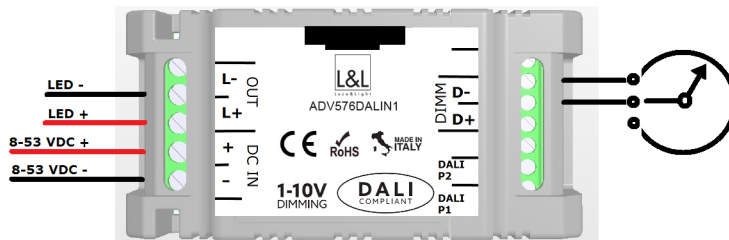
Collegamento potenziometro (fig. 3) / Potentiometer connection (pic. 3)
