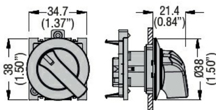
Long lever
