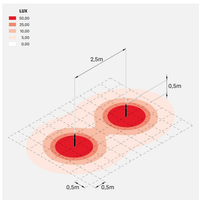
stik_60_trasp_500_6w
