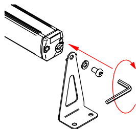
INSTALLAZIONE INTERNA INTERNAL INSTALLATION
