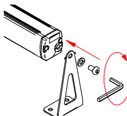
INSTALLAZIONE ESTERNA EXTERNAL INSTALLATION
