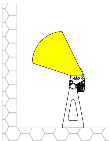
5A) INSTALLAZIONE A PAVIMENTO FLOOR INSTALLATION
