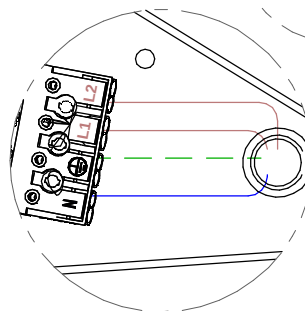
DETTAGLIO T DETAIL T
