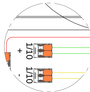
DETTAGLIO G DETAIL G
