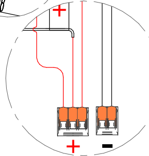
DETTAGLIO V DETAIL V
