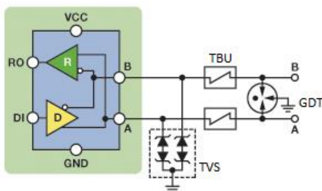
Figura 2: Configurazione della protezione per la porta DMX IN - Configuration of protection for the DMX IN port.
