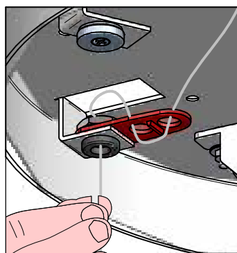
DETTAGLIO A
