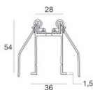
Controcassa posizione installativa: pavimento; tipo installazione: cartongesso L=510mm, H=55.5mm, D=36mm. Materiale:alluminio, colore:Anodised aluminium, lavorazione:anodizzazione.
