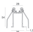
Einbaugehäuse
