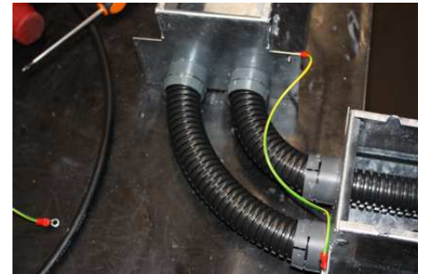
ESEMPIO CURVA A 90° - 90° CURVE EXAMPLE
