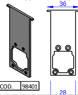
Accessorio (5) - Accessory (5)
