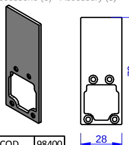
Accessorio (8) - Accessory (8)
