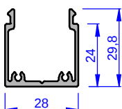
Accessorio (5) - Accessory (5)
