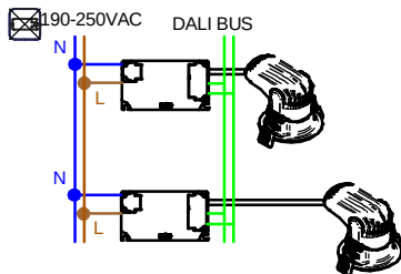
COLLEGAMENTO SINGOLO DALI SINGLE CONNECTION DALI
