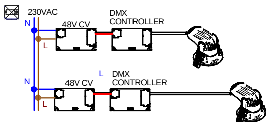
COLLEGAMENTO SINGOLO DMX BIANCO DINAMICO SINGLE CONNECTION DMX DYNAMIC WHITE
