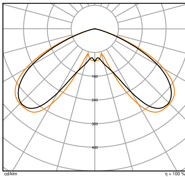
URBAN VLA P 40W 730 SYM140
