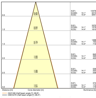
UB WL VARIO SQ 29W ML 830 GY 30D Down
