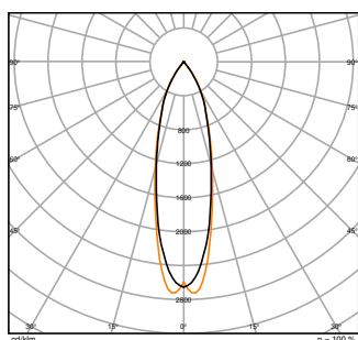
UB WL VARIO SQ 29W ML 840 GY 30D Down
