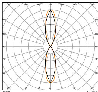
UB WL VARIO RD 29W ML 827 GY 30D Up Down
