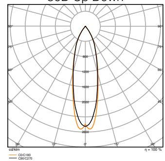
UB WL VARIO RD 29W ML 822 GY 30D Down
