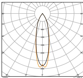
UB WL VARIO RD 29W ML 827 GY 30D Down
