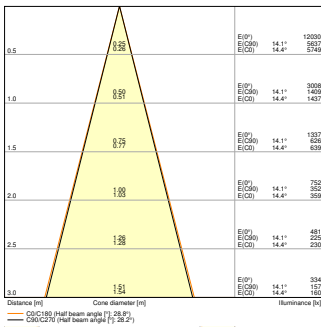
UB WL VARIO RD 29W ML 822 GY 30D Down
