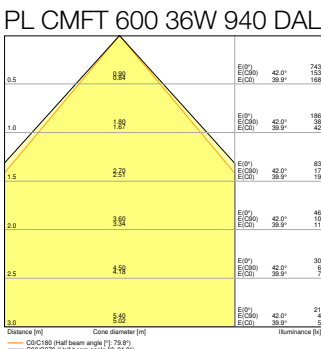
PL CMFT 600 36W 940 DALI EM mode
