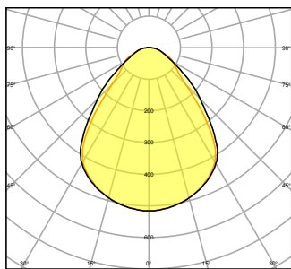
PL CMFT 600 36W 930 DALI EM mode
