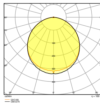
PL CMFT 1200 33W 840 PS EM CONVERSION BOX
